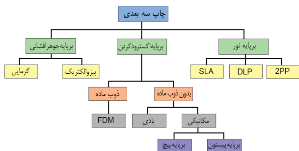
شکل ۱- طرحی از دسته‌بندی انواع فناوری‌های چاپ سه بعدی [۹].
