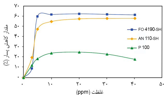
شکل ۹- مقایسه پلیمرهای آنیونی، کاتیونی و غیریونی در غلظت‌های مختلف با چگالی بار یکسان [۱۳].
