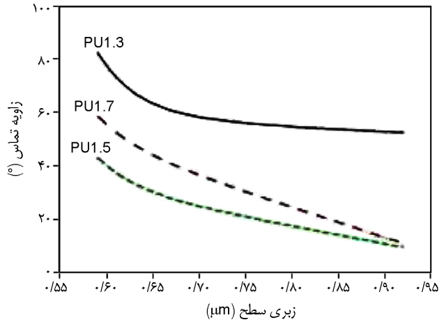
شکل ۶- اثر زبری سطح بر ترشوندگی [۱۹].
