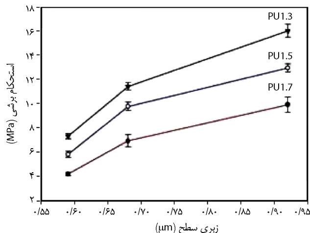
شکل ۷- اثر زبری سطح بر استحکام چسبندگی برشی [۱۹].
